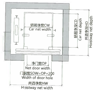
井道平面布置图
