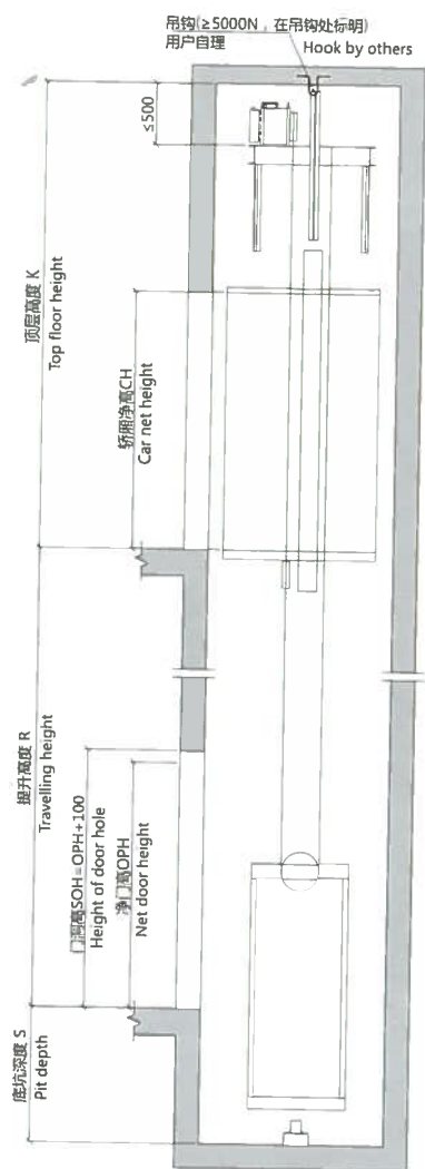
Hoistway elevation
